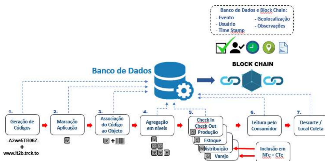
Figura 1: Arquitetura genérica do módulo de Block Chain
